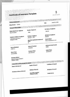
Deskew
